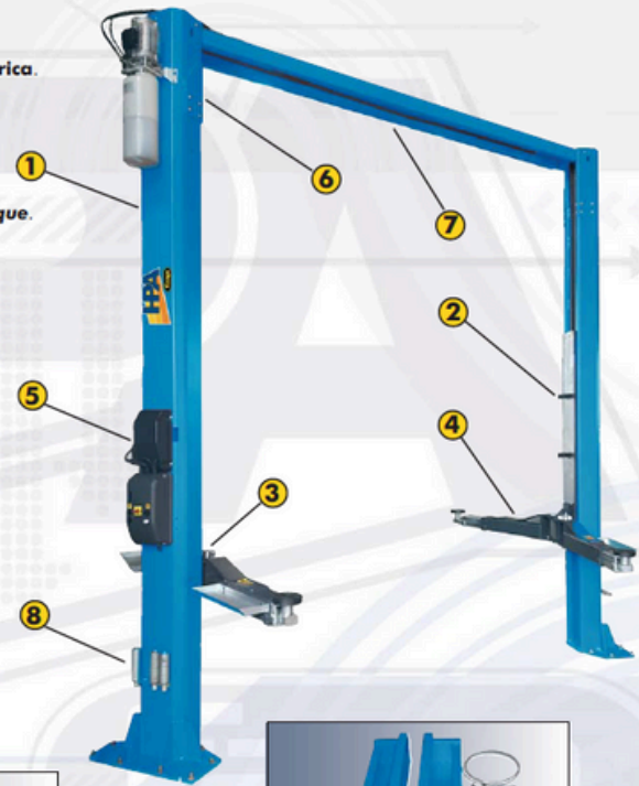
5. Sblocco sicuro con elettromagnete 24V Sécurité mécanique à déverrouillage automatique par électroaimant 24 volts.
