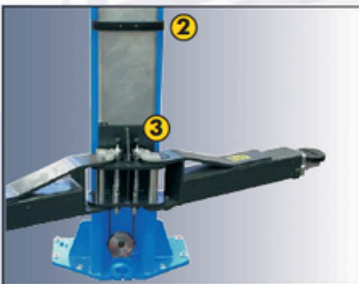
2. Protezioni in gomma salvaportiera. Bande en caoutchouc pour protéger les portières. 3. Arresto rotazione bracci a settori dentati Système automatique de blocage des bras avec roues crantées.
